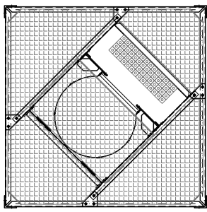
sez. A-A
