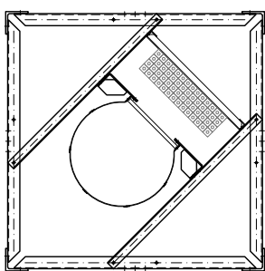
sez. I-I
