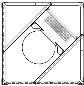
sez. D-D
