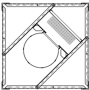
sez. H-H
